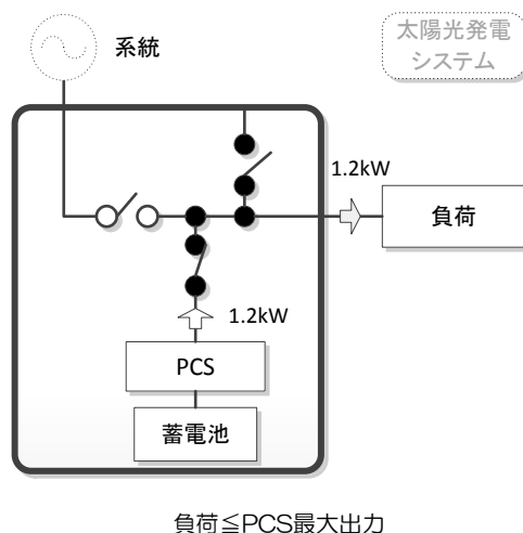
図 22：単体設置時の動作イメージ(停電モード)
