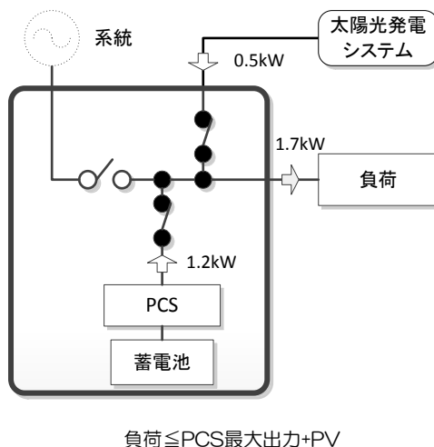
図 23：太陽光発電システム接続時の動作イメージ（停電モード時）
