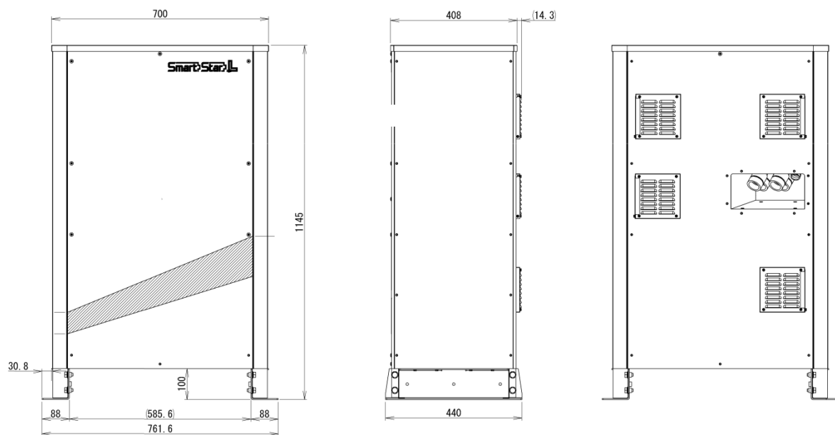
図 25 : 外形寸法図(本体)
