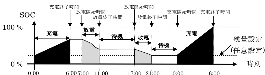
図 5：充放電動作イメージ
