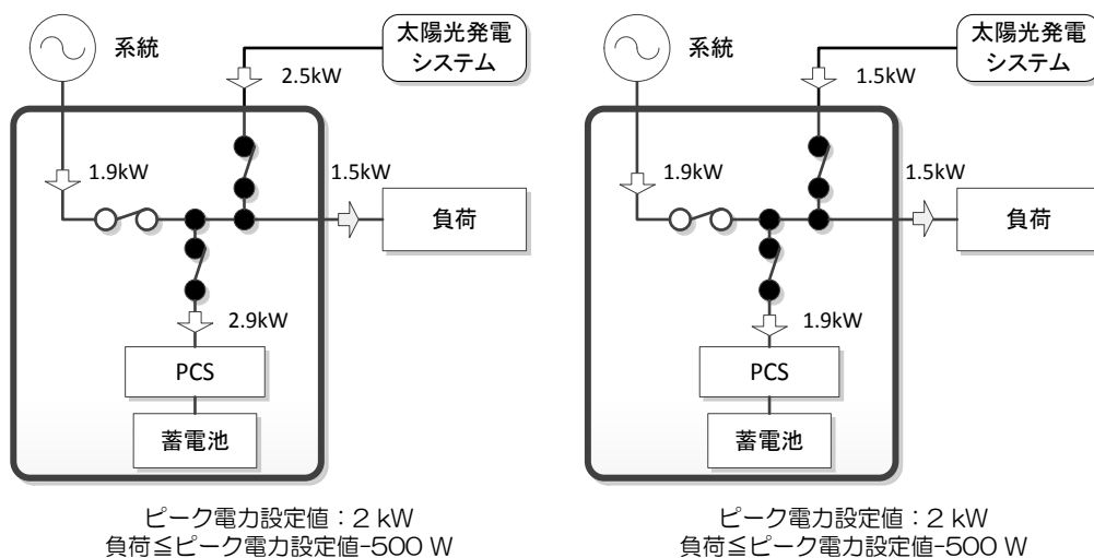
図 11：太陽光発電システム接続時の充電動作イメージ(ピークカットモード)
