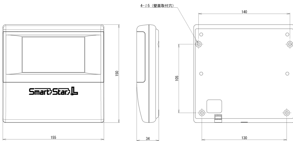
図 26 : 外形寸法図(エネルギーモニター)
