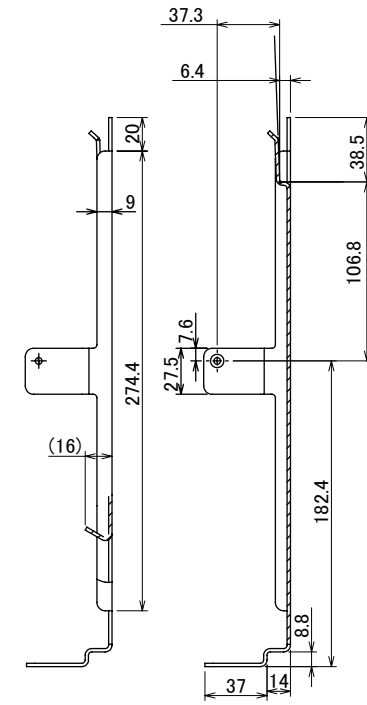
断面図 A-A
